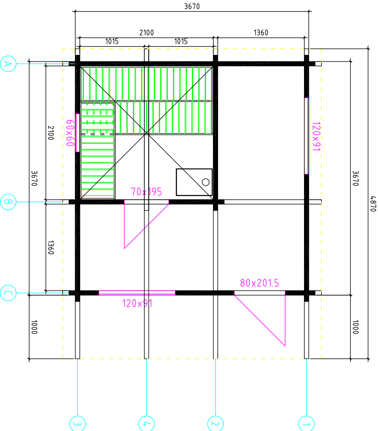
Grundplan
