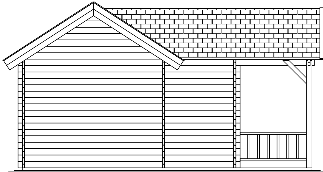
zijaanzicht (I) / side view (I)
