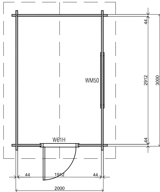
Plattegrond / Plan
