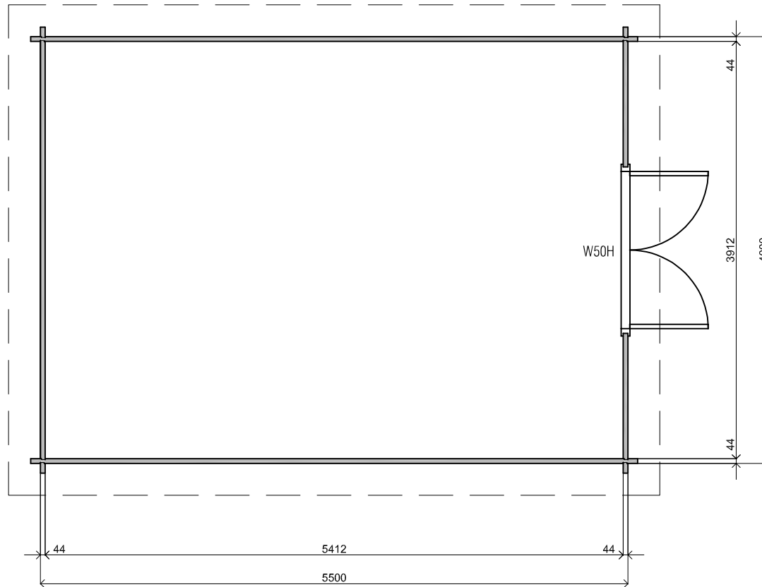
Plattegrond / Plan
