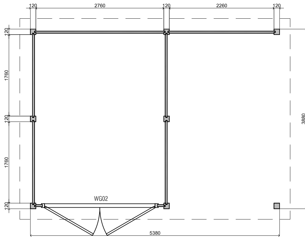
Plattegrond / Plan
